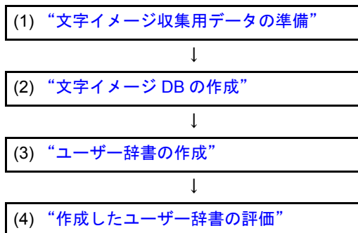
図 13.1 ユーザー辞書の作成の流れ
