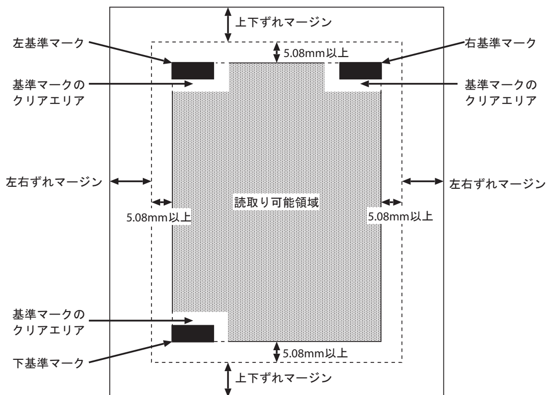
図 C.20 基準マーク
