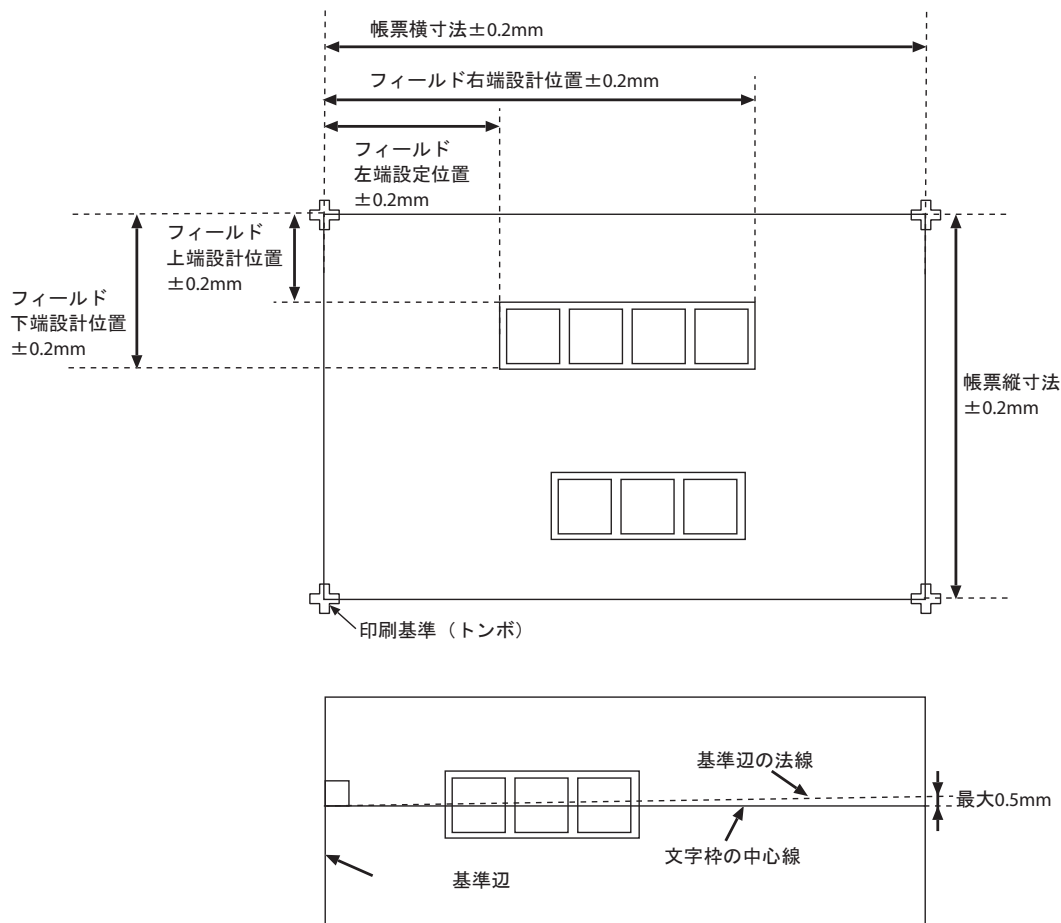
図 C.18 印刷精度
