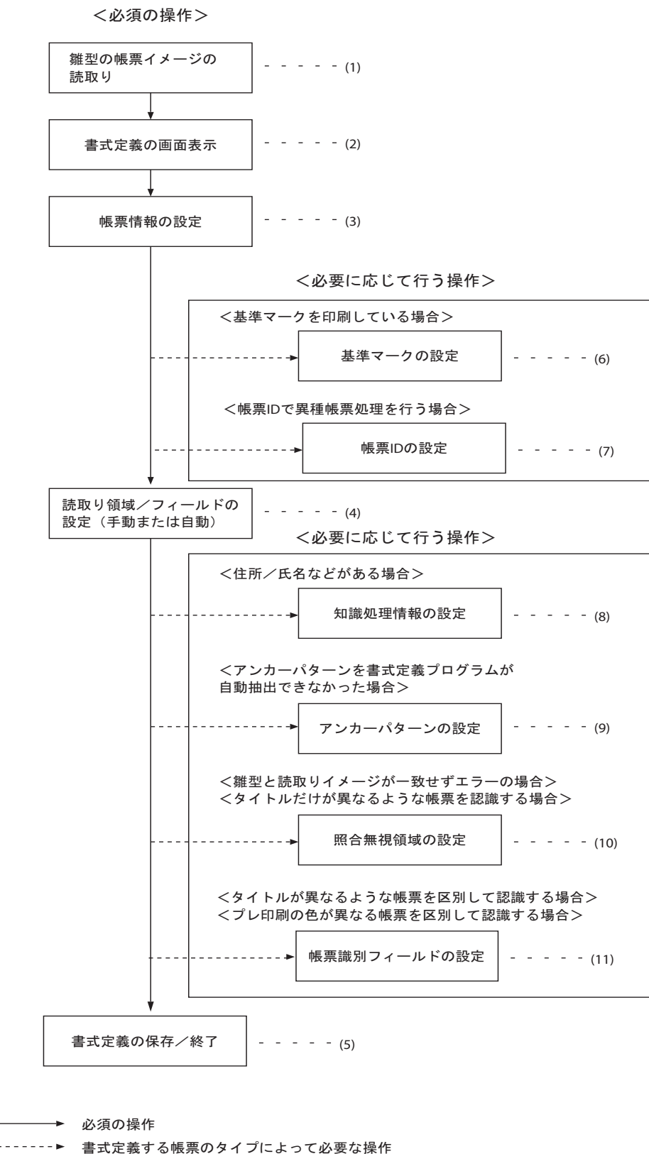
図 8.1 書式定義を行う手順
