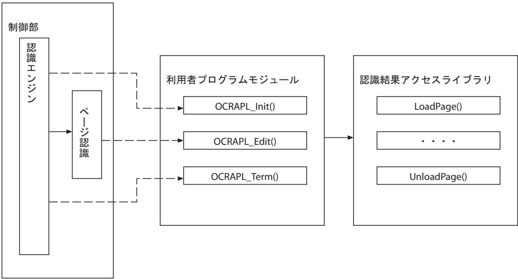
図 1.1 モジュール構成図
