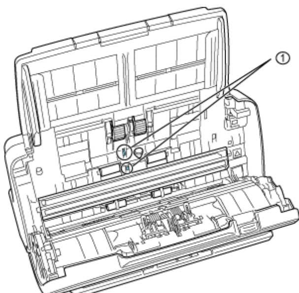
原稿検知センサー
