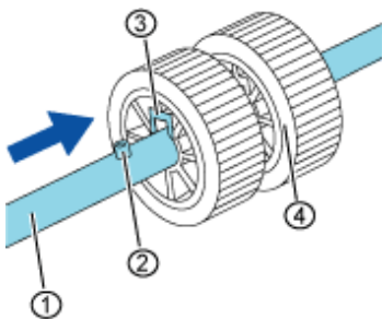
ピックローラ軸 突起 溝 ピックローラ
